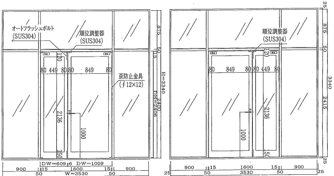
室外側立面図
