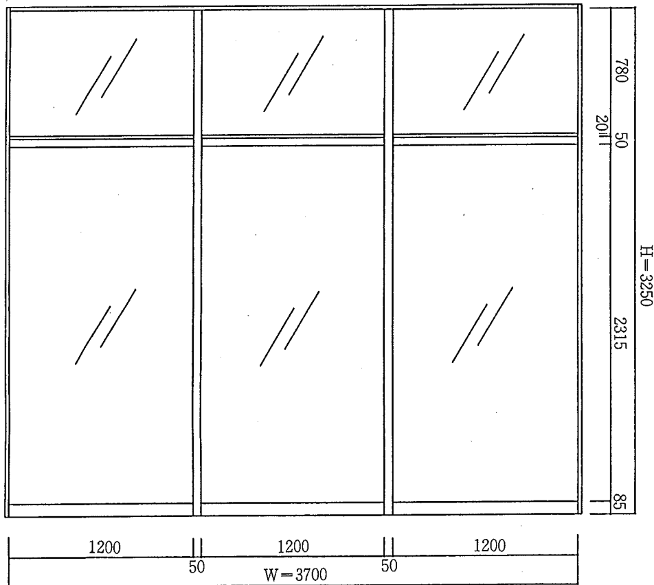
室外側立面図
