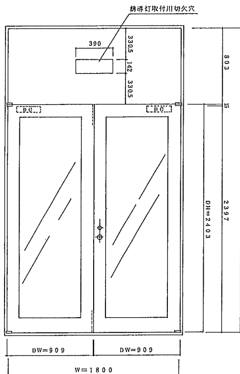
屋外側立面図
