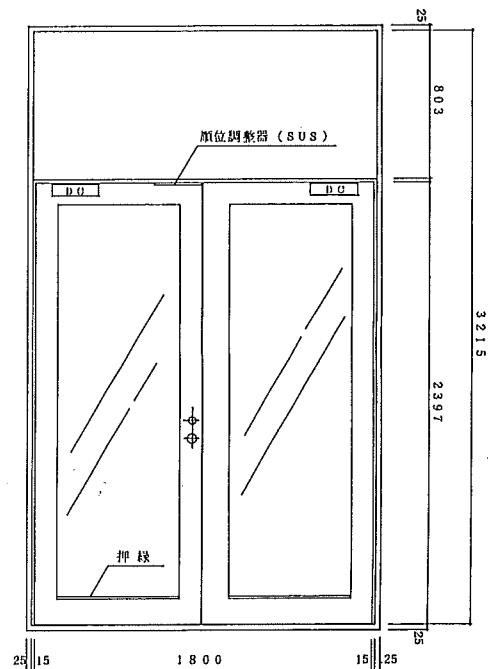
屋内側立面図
