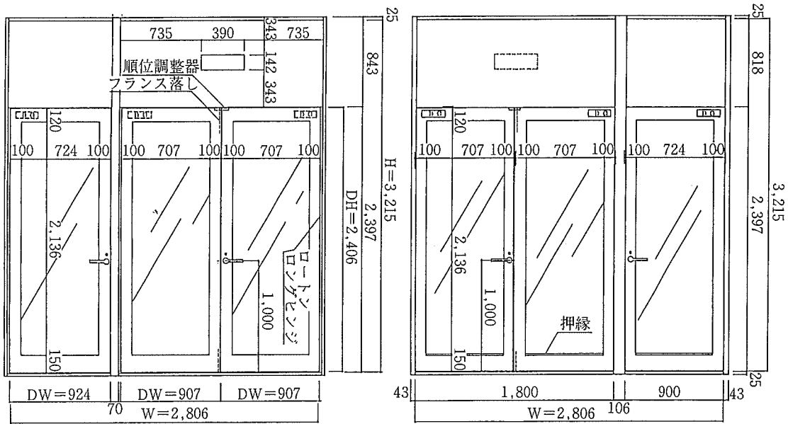
室外側立面図
