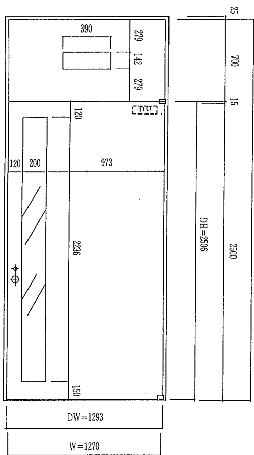
屋外側立面図
