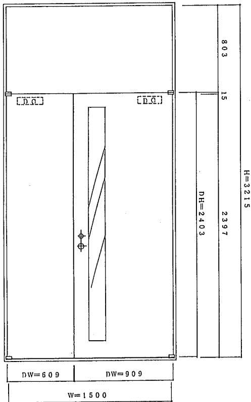
屋外側立面図
