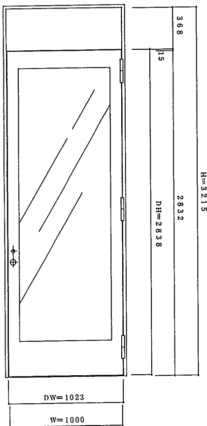
外側立面図
