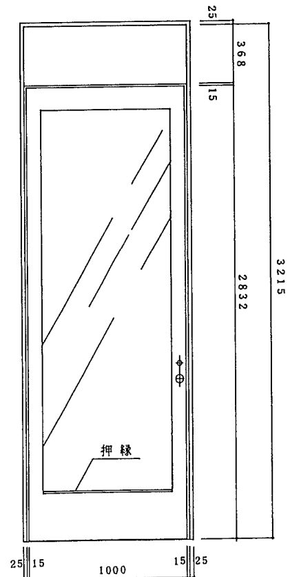
屋内外立面図
