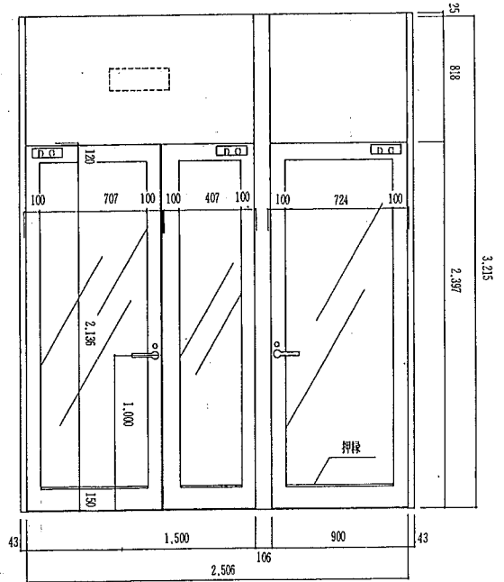
室内側立面図
