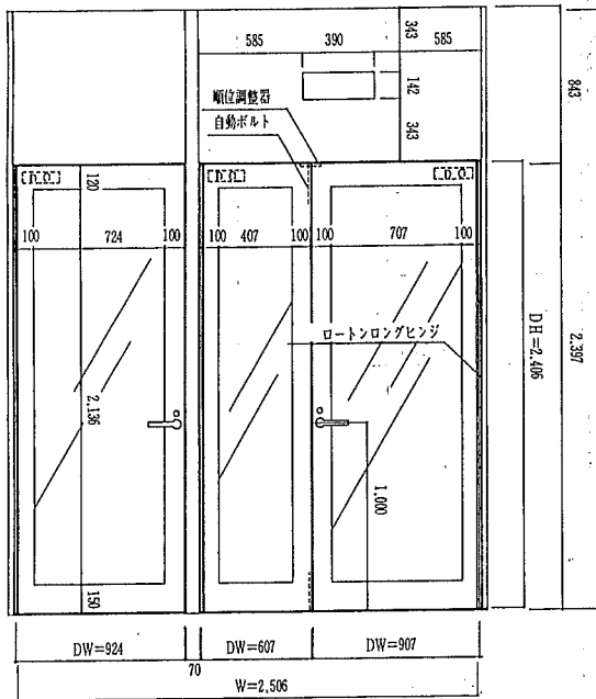
室外側立面図
