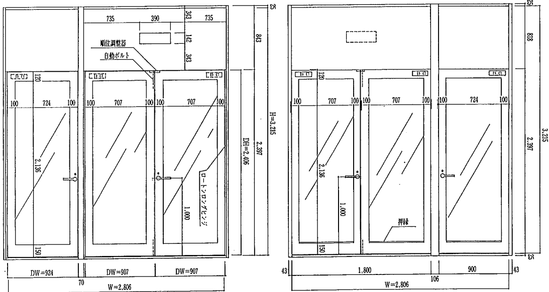
室内側立面図
