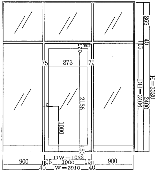
室外側立面図
