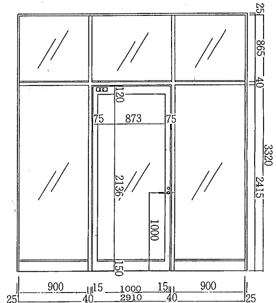
室内側立面図
